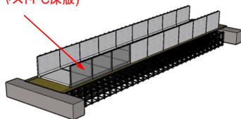
下床版パネル設置
