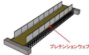
底版組立・プレテンションウェブ建込
