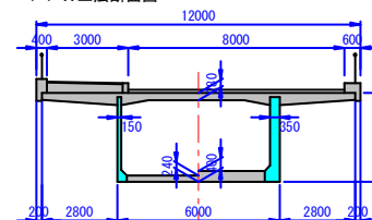
支間中央 支点上
