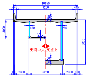
PPW工法断面図
