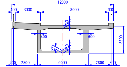
従来工法断面図
