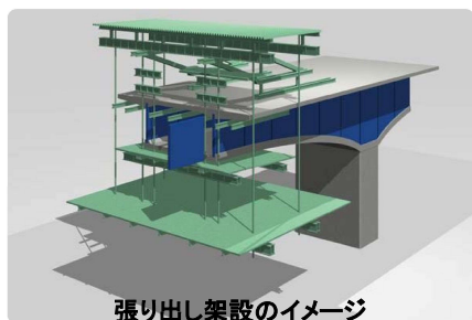
張り出し架設のイメージ
