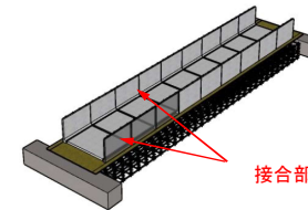
上床版接合・外ケーブル緊張・支保工解体
