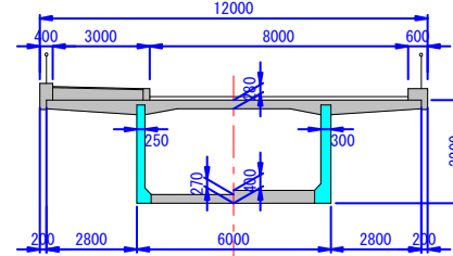
PPW工法断面図
