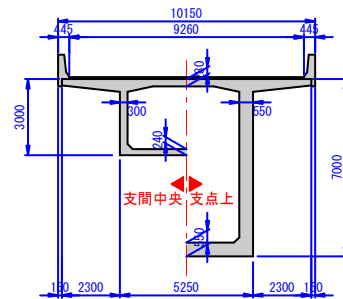
従来工法断面図
